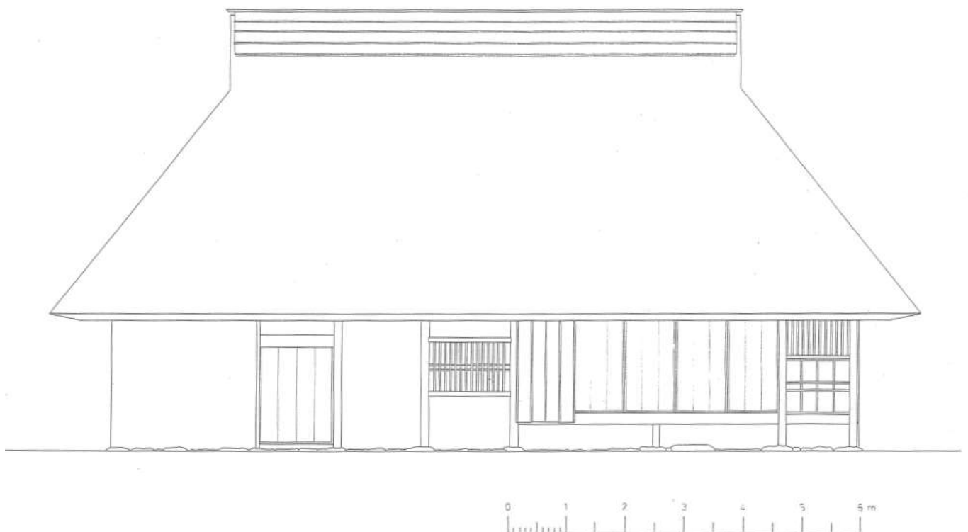
旧河野家 立面図側面（西面）（東面）
