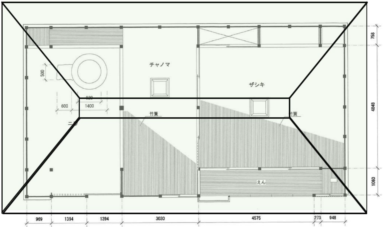
旧河野家 屋根俯瞰図
